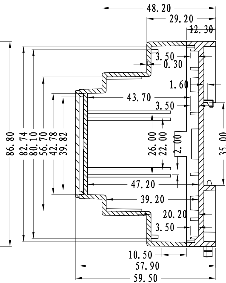
SEC A-A
