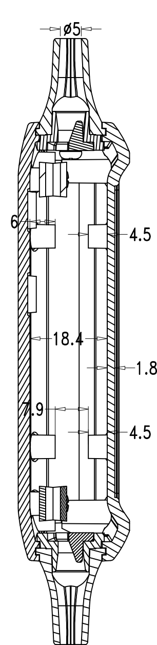
SEC A-A
