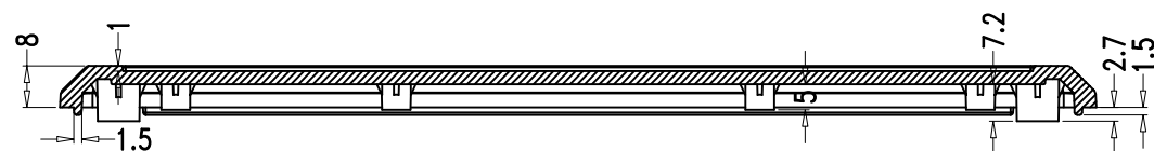
SEC A-A
