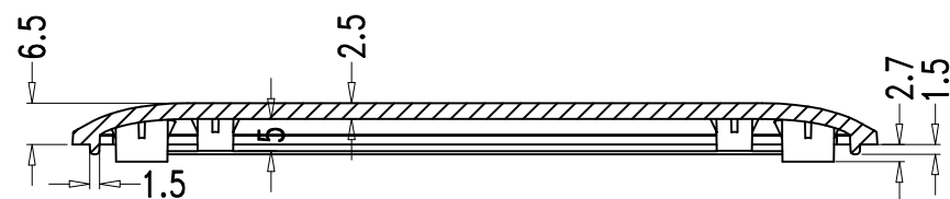
SEC A-A
