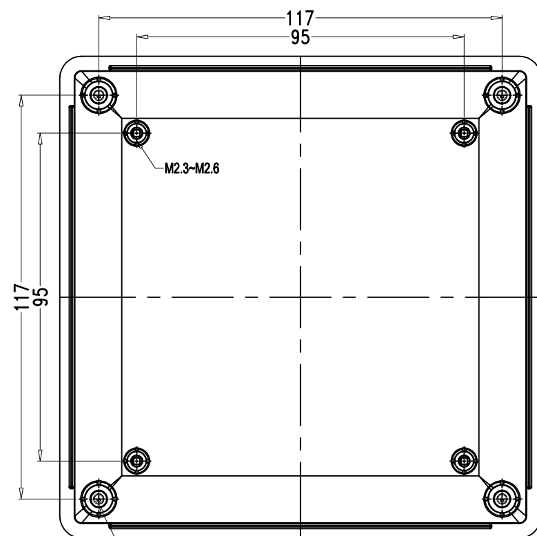
SEC A-A
