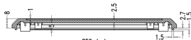
SEC A-A
