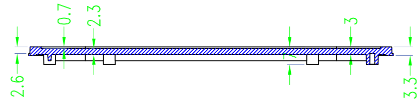
SEC A-A
