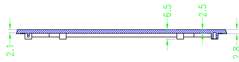
SEC A-A
