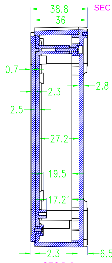
SEC D-D
