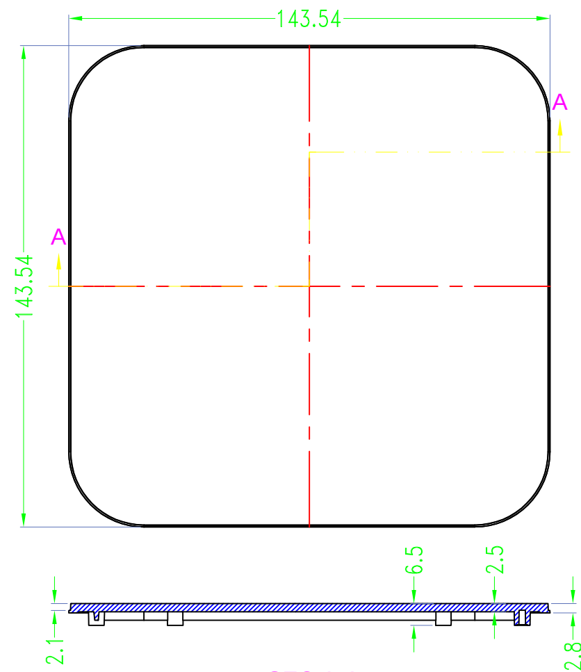
SEC A-A
